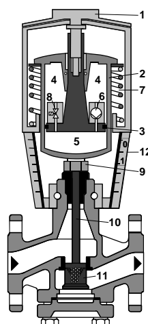
Клапан открыт
