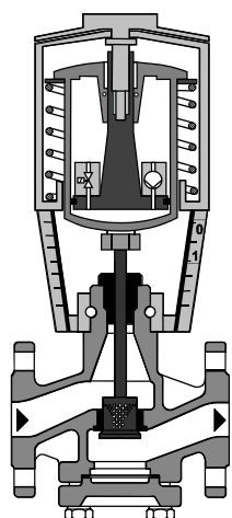
Клапан закрыт
